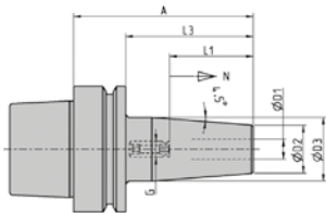
T... HSK-E32, DIN 69893 Shrink chuck
