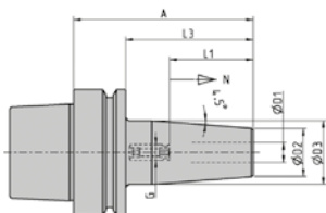
T... HSK-E40, DIN 69893 Shrink chuck
